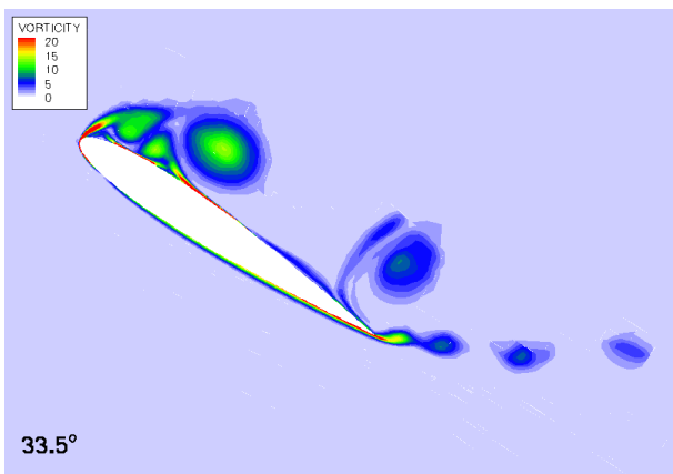
(d) vortices grow
