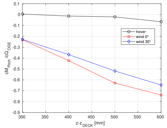
(d) Pitch moment coefficient, vertical landing
