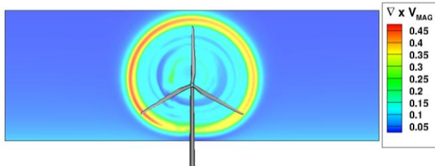
b) Vorticity field
